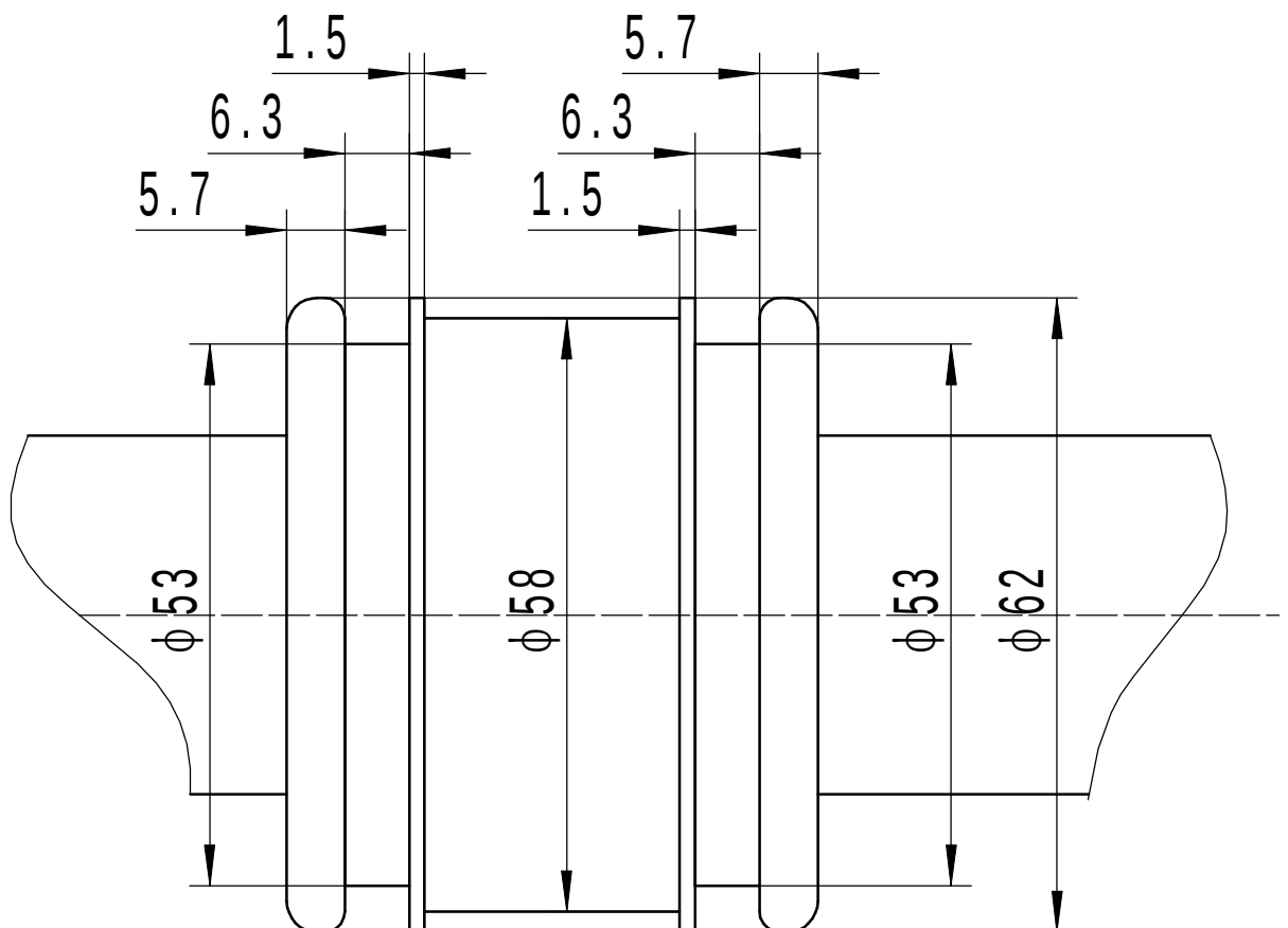
活塞及油封槽测量尺寸
