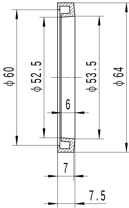
油封形状及测量尺寸
