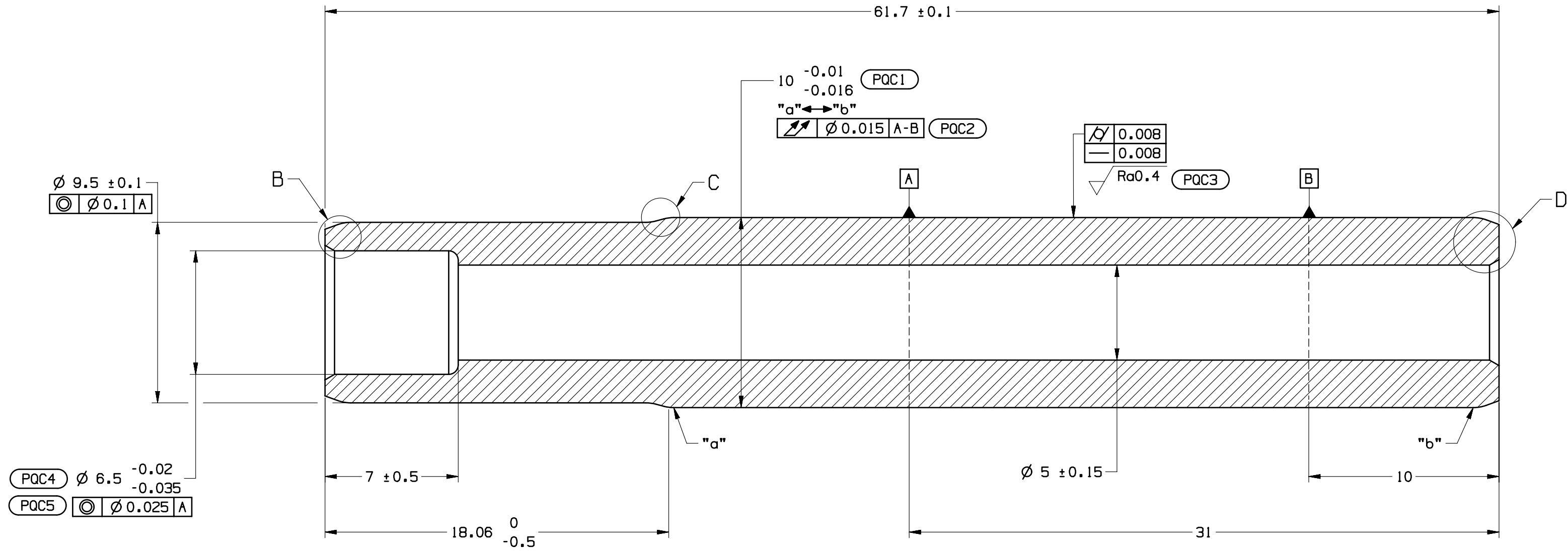
SECTION A-A
