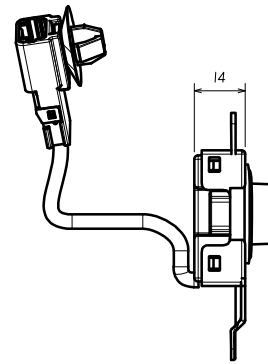
正视图 缩放: 1
