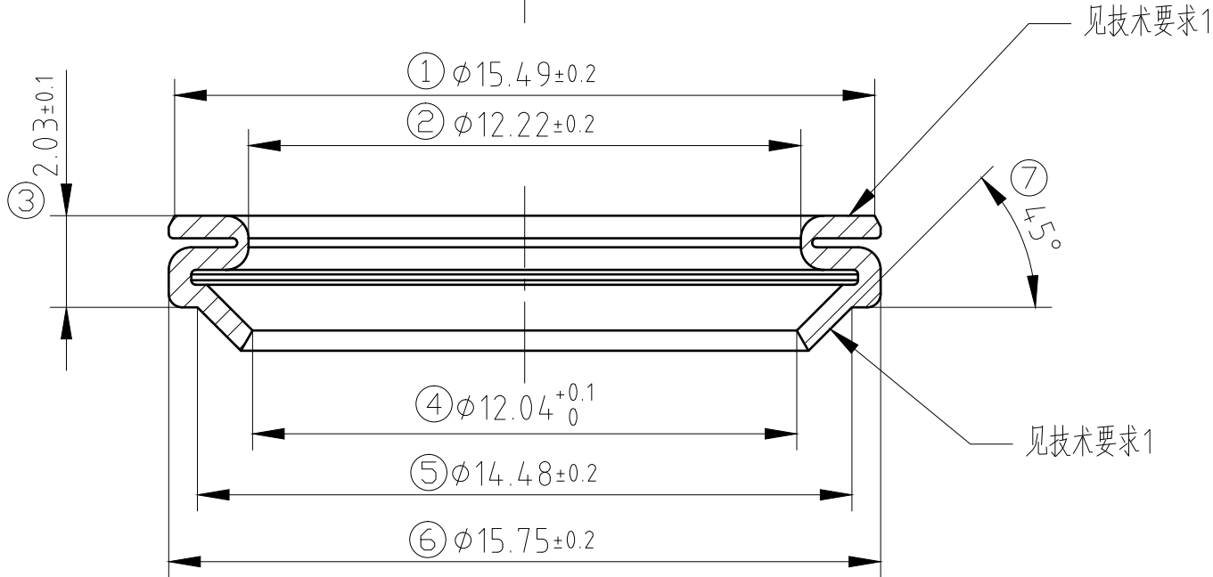
截面 A - A
